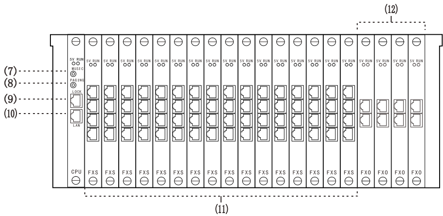
D256K 后视图:
